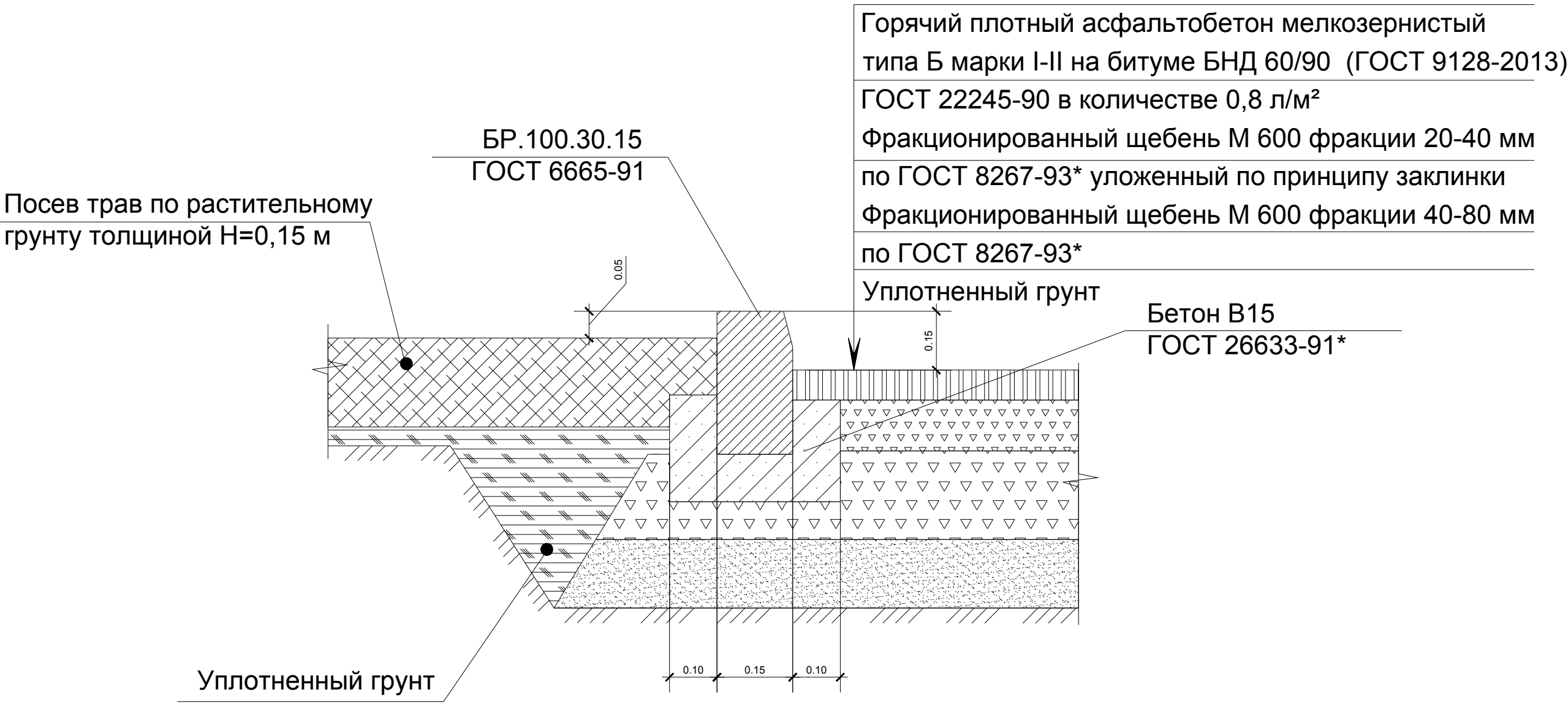
Конструкция покрытия с тактильной плиткой
