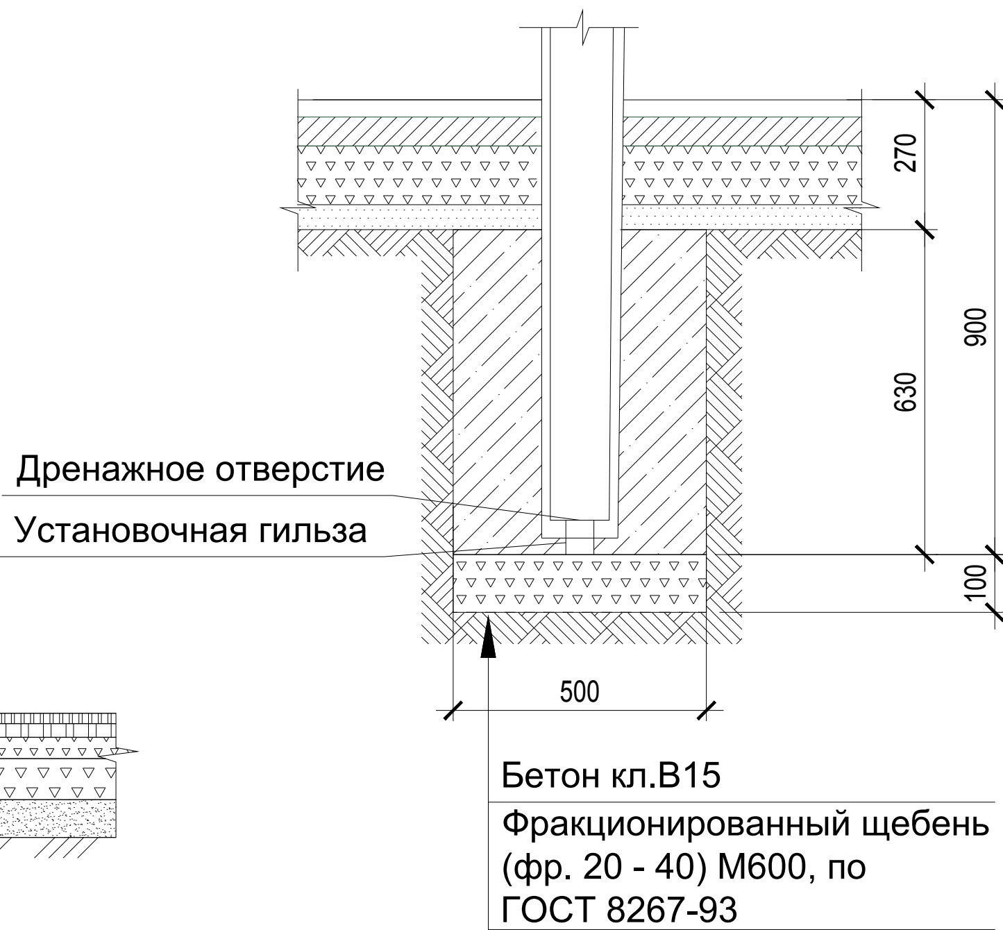
Узел устройства фундамента стойки МАФ
